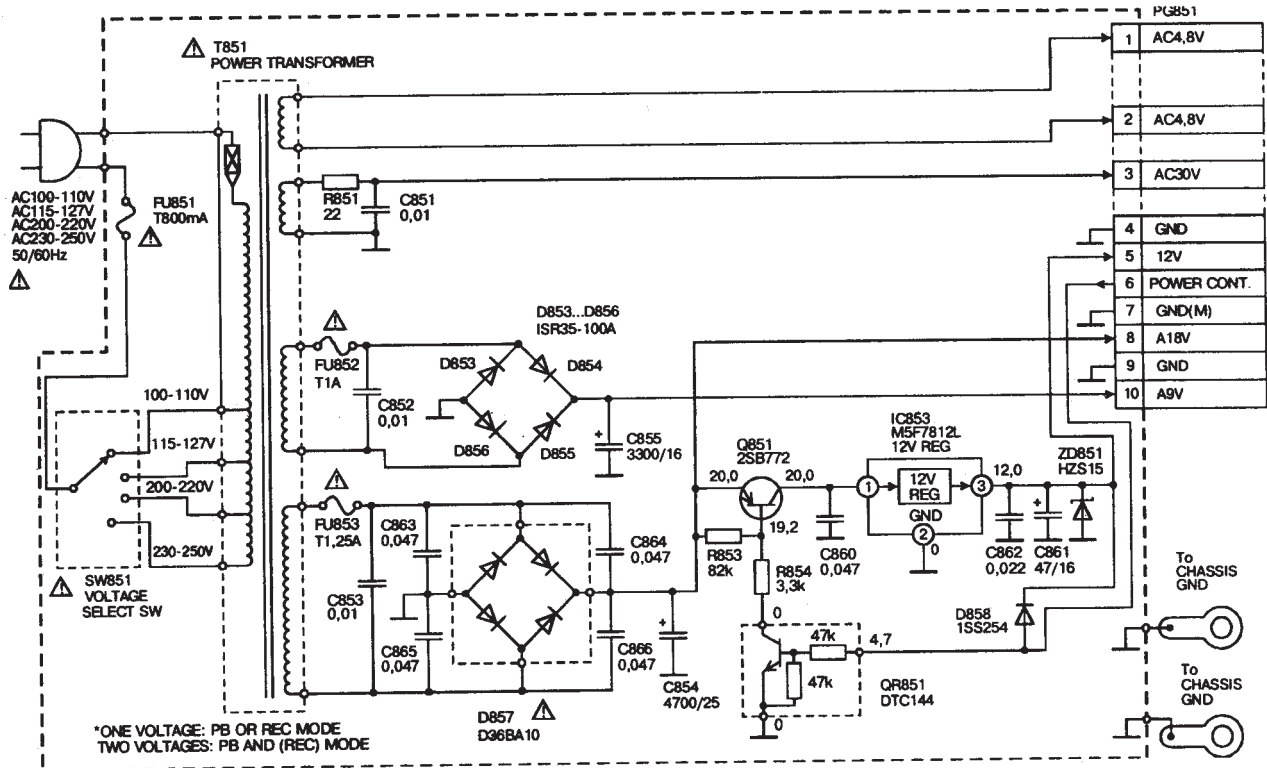
Принципиальная схема источника питания видеомэагнитофона VT-M619EM.
